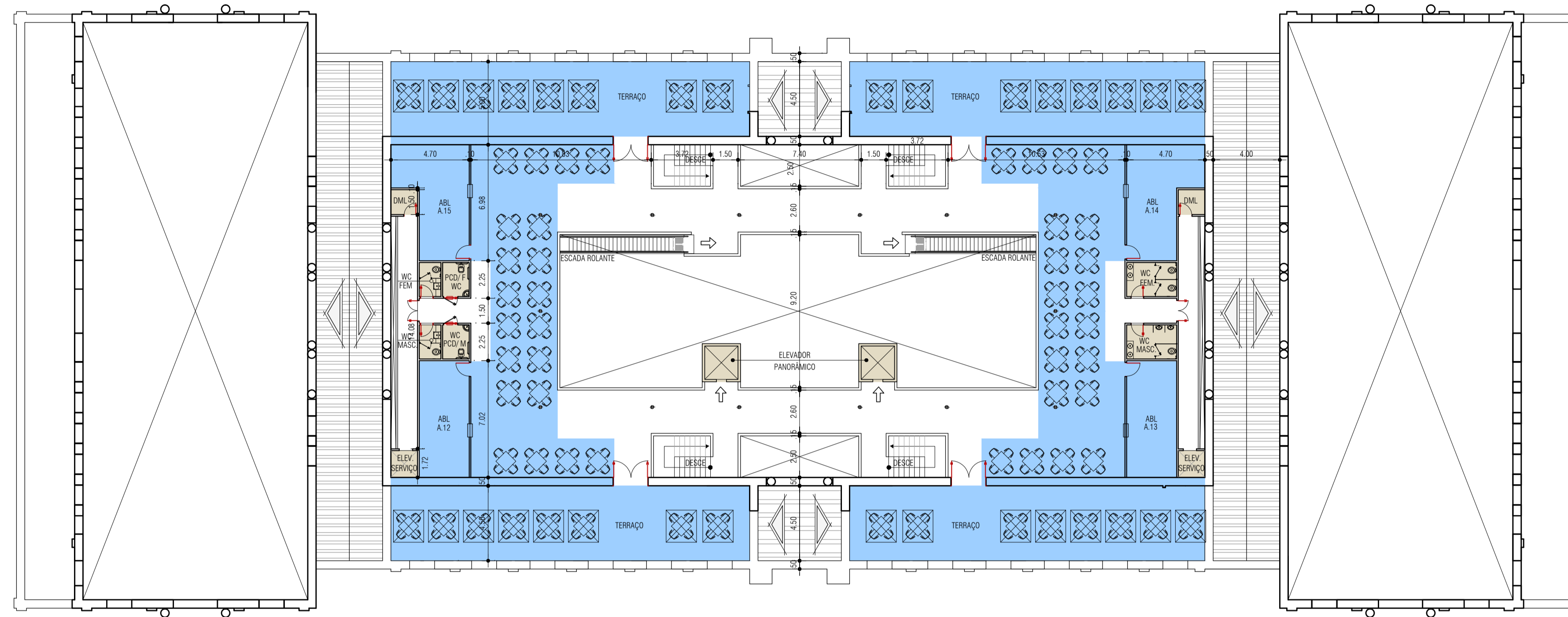
MEZANINO 2 ESCALA: 1/200
